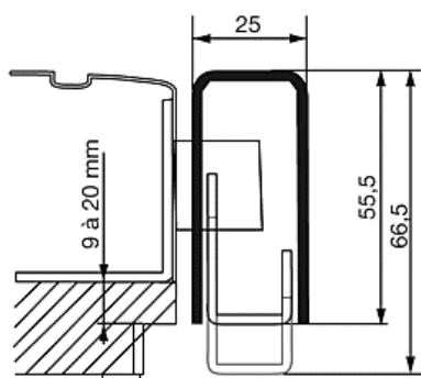
Gâche GAR pour porte à recouvrement de 9 à 20 mm
