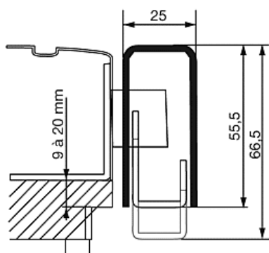
Gâche GAR pour porte à recouvrement de 9 à 20 mm
