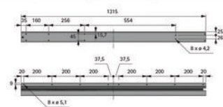
Dimensions de planification longueur de montage 1315 mm
