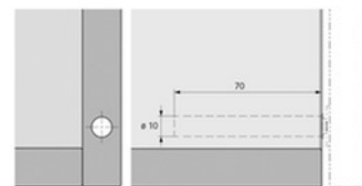
Schéma de perçage pour course longue, porte en applique
