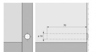
Schéma de perçage pour course longue, porte en applique
