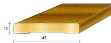
Section du couvre joint
