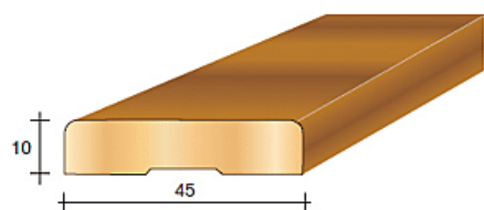
Section du couvre-joint
