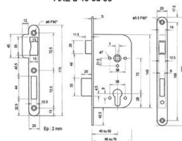
SERRURE 667 NF AXE à 40 ou 50
