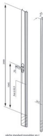
gâche standard monobloc en Z
