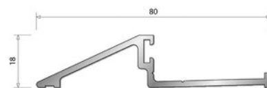
Coupe verticale sur ouvrant
