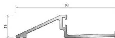
Coupe verticale sur ouvrant
