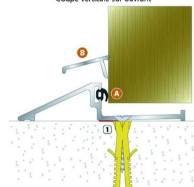
Coupe verticale sur ouvrant
