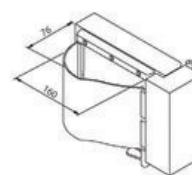
Encombrement APD sur porte bois standard
