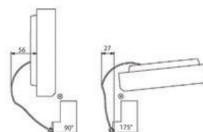
Encombrement APD sur porte bois standard
