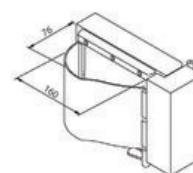
Encombrement APD sur porte bois standard
