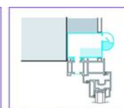
Montage en haut de fenêtre
